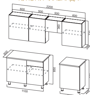
КУХНЯ 2,2 М
