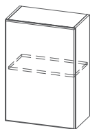
Ш200/Ш300/Ш350/Ш400/ Ш450/Ш500/Ш600 (1 СТБ.) 200/300/350/400/450/ 500/600x720x296 мм
