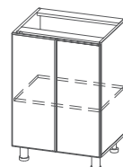
С550/С600/ С700/С800 550/600/700/ 800x824x506 мм
