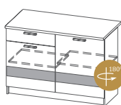
Стол под мойку 1200* 1200x850x448 мм
