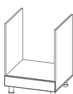
С600п 600x824x538 мм
