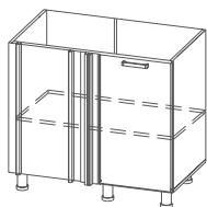
C1000y* 900x824x506мм
