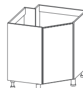
M850y 790x824x790мм
