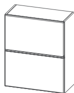
Ш400б/Ш600б/Ш800б 400/600/800x720x296 мм
