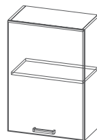
Ш300/Ш400/Ш500 300/400/500x720x296мм
