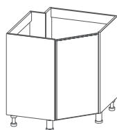
M850у* 790x824x790мм
