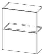
Ш500б/Ш600б/Ш700б/ Ш800б (Aventos HF)*7 500/600/700/800x720x296 мм
