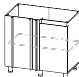
С1000у 900x824x540 мм (1000 угловой правый)
