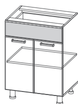
М600/М800* 600/800x824x506мм
