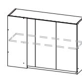
Ш1000у 1000x720x296 мм (1000 угловой правый)
