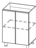
M600/M800* 600/800x824x506мм
