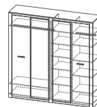
Шкаф для платья и белья четырёхств-й 2160x2200x545 мм
