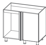
М1000у 900x824x506 мм
