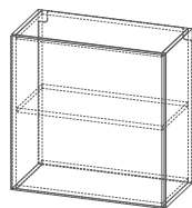
ШГ600x600 600x600x296 мм
