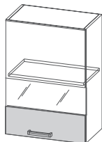
Ш300с/Ш400с/Ш500с 300/400/500x720x296мм
