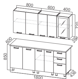
КУХНЯ 1,8 М
