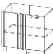
C1000у* 900x824x506мм
