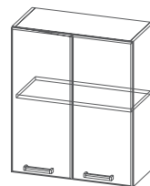
Ш600/Ш800 600/800x720x296мм
