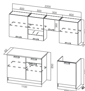
КУХНЯ 2,2 М
