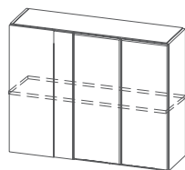
Ш1000у*5 1000x720x296 мм
