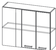
Ш1000у 1000x720x296мм
