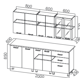
КУХНЯ 2,0 М
