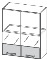
Ш600с/Ш800с 600/800x720x296мм
