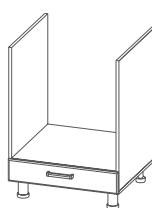
С600п* 600x824x538мм
